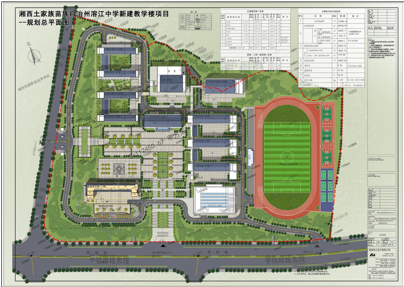
总平面图
