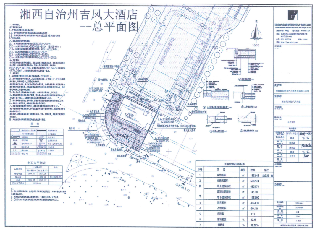
调整后总平面图
