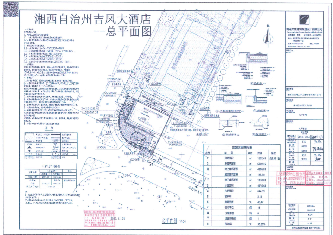
调整前总平面图
