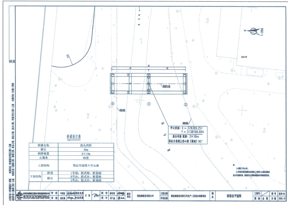
平面图
