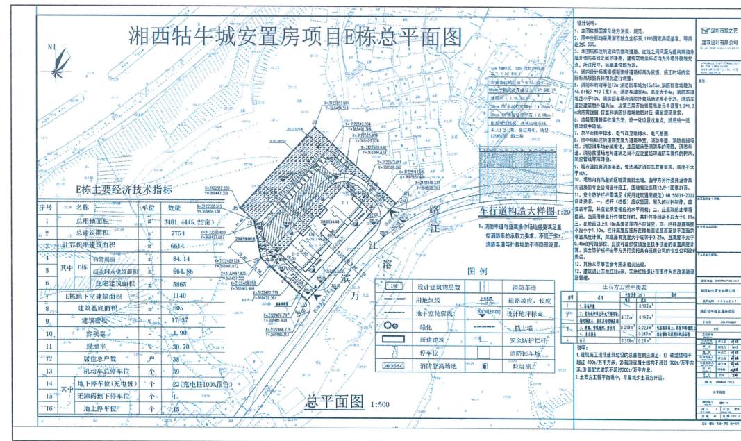
变更后总平面图
