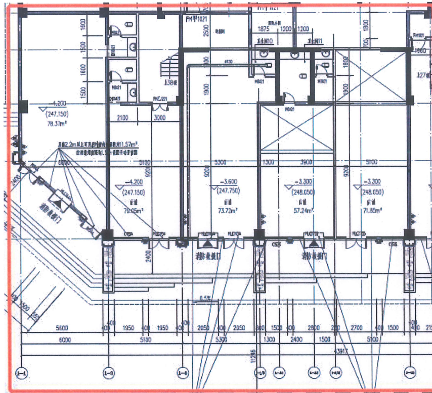
负一层平面图
