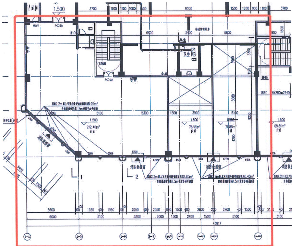
一层平面图
